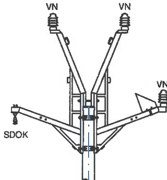
aplikace - alt.1 - Optický kabel vlevo
