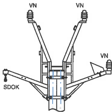
aplikace - alt.2 - Optický kabel vlevo
