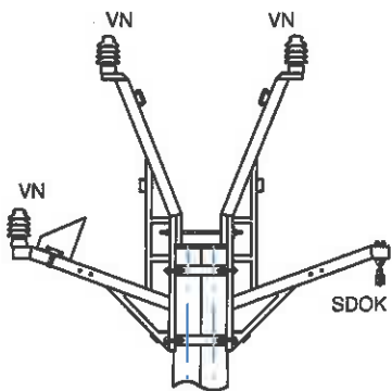
aplikace - alt.1 - Optický kabel vpravo
